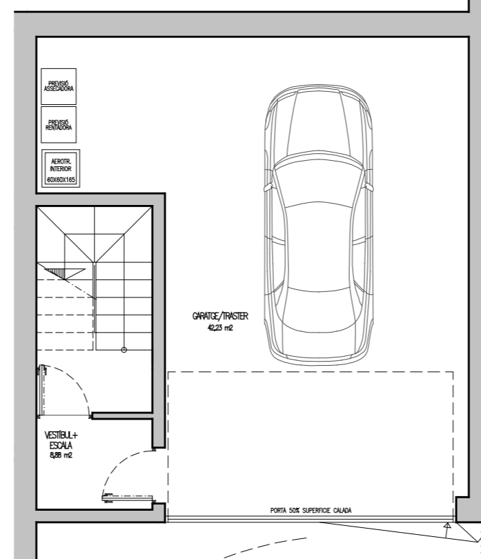
Planta Soterrani
