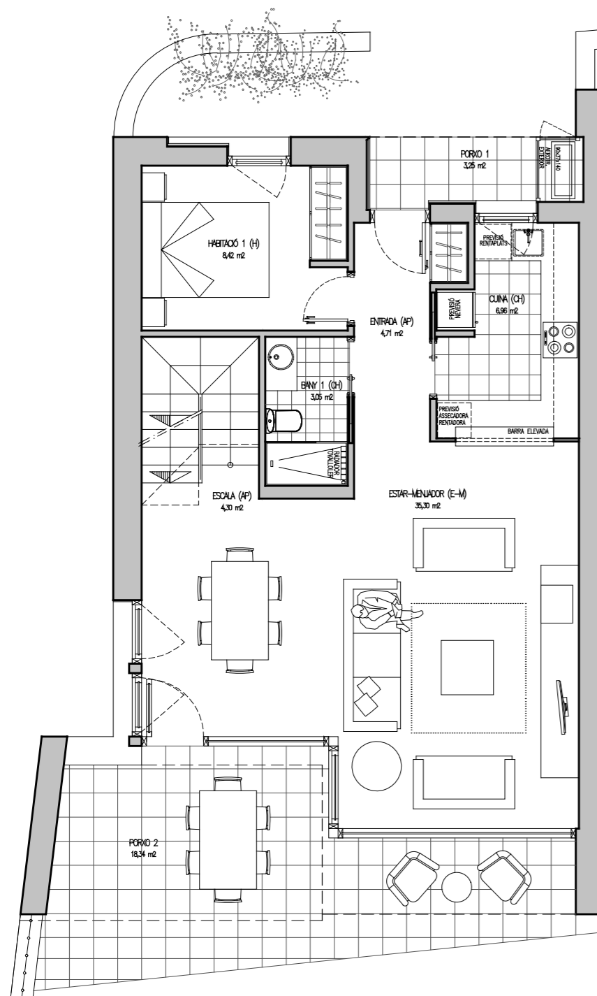
Planta Baixa
